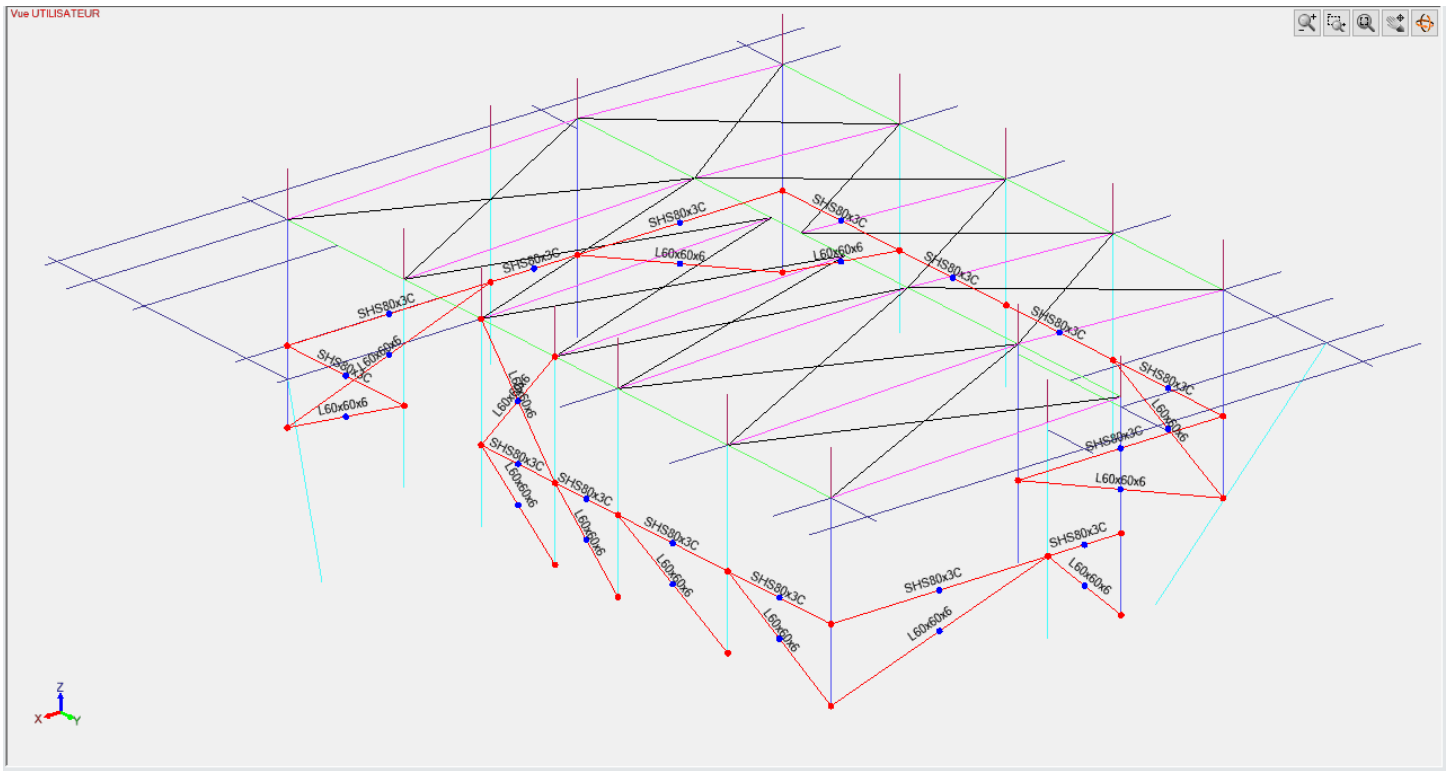
Lisses et stabilités verticales
