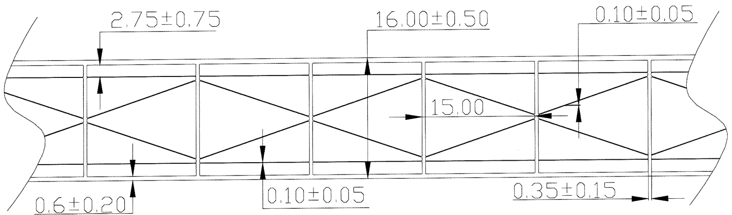
Figure 4 : Coupe type des vitrages organiques multiparois « Quinn SPC » en 16mm d'épaisseur, 3 parois (cotations en mm)
