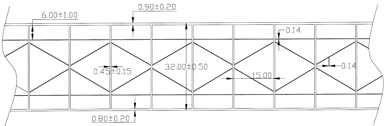
Figure 5 : Coupe type des vitrages organiques multiparois « Quinn SPC » (cotations en mm)
