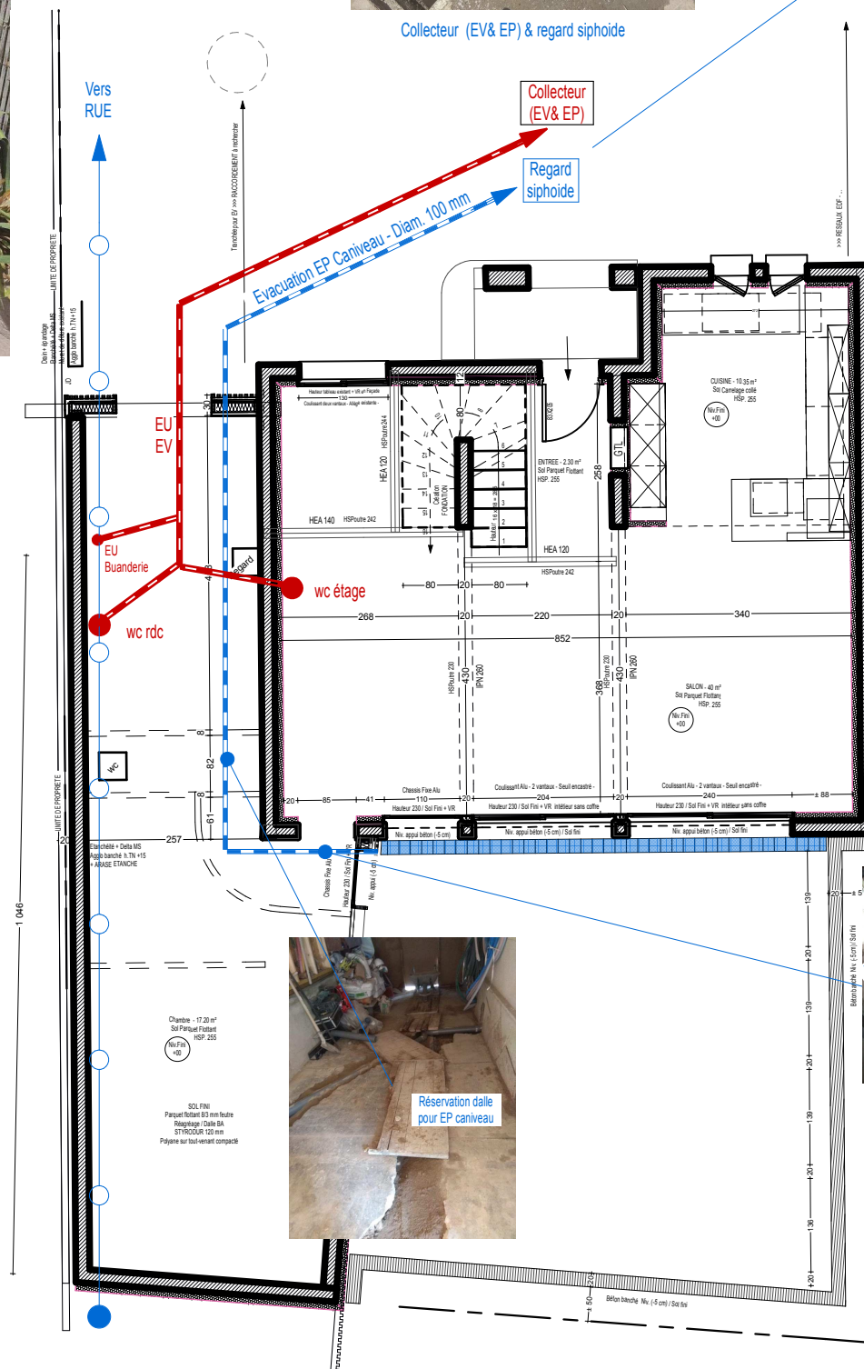
Collecteur (EV&EP) avant la pose du regard siphoine
